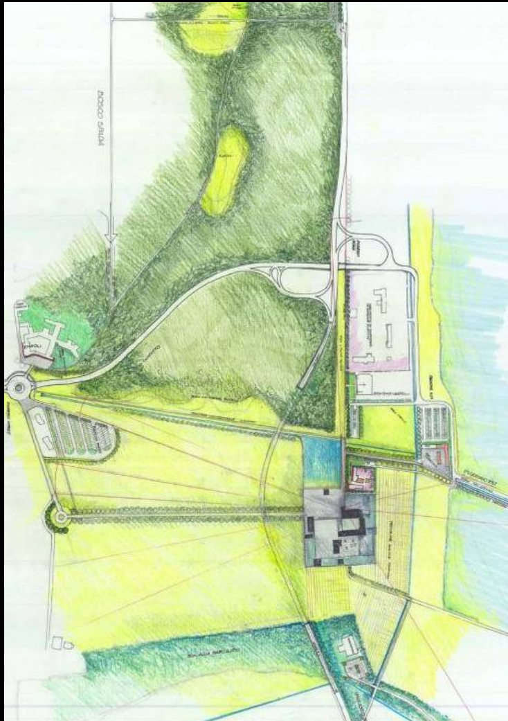
schizzo progettuale
